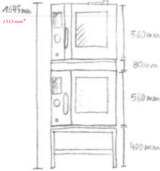
Station CombiMix avec JOKER et panneau de commande sur le côté sur un support de 400 mm.
