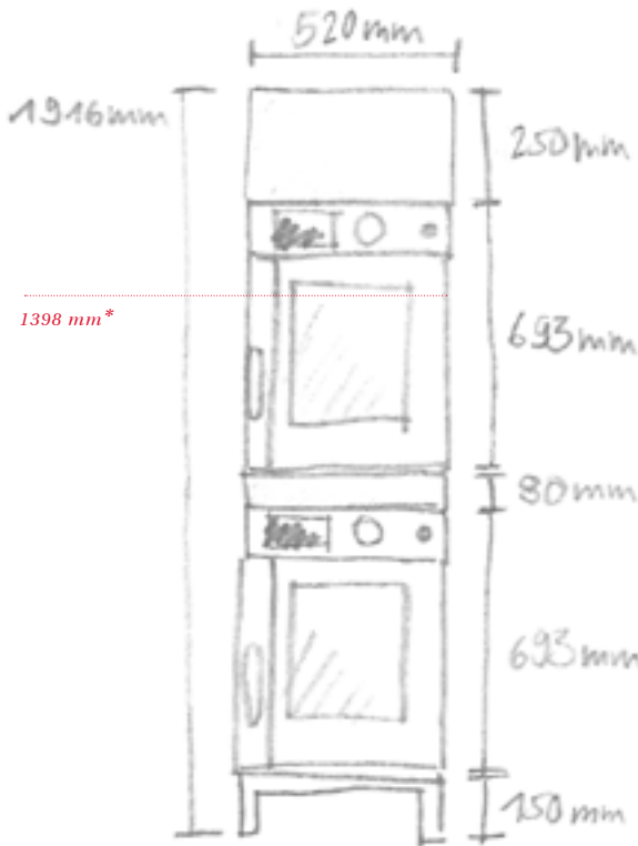
Station CombiMix avec JOKER et panneau de commande sur le dessus avec KH1 sur un support de 150 mm.
