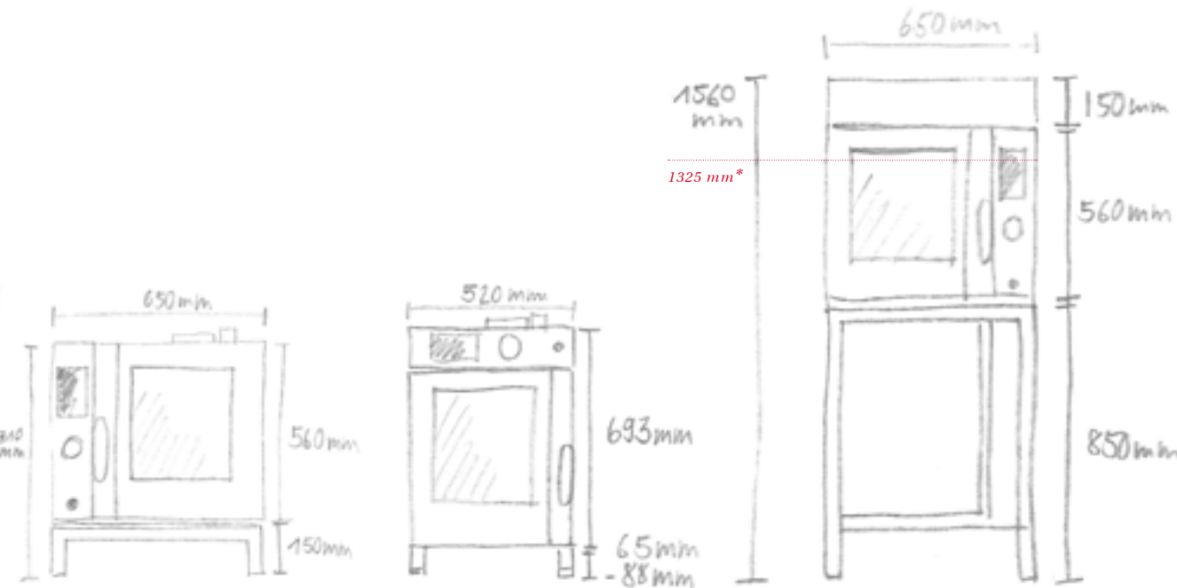
JOKER avec panneau de commande sur le côté sur un support de 150 mm.
